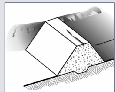
Longitudinal Crack
